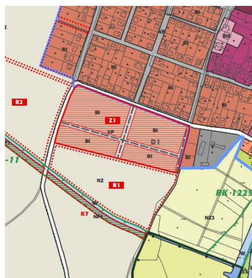
Obrázek 5 Výkres územního plánování Rožďalovic, zdroj: (Město Rožďalovice, 2018)
